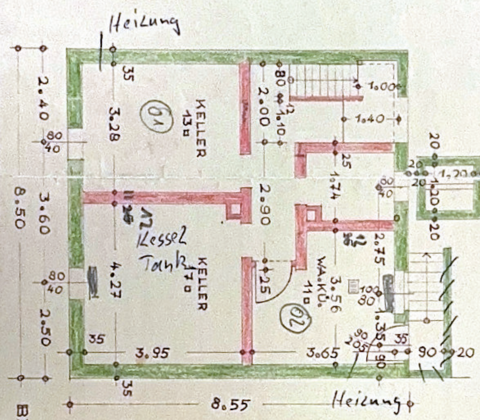
SCHNITT
