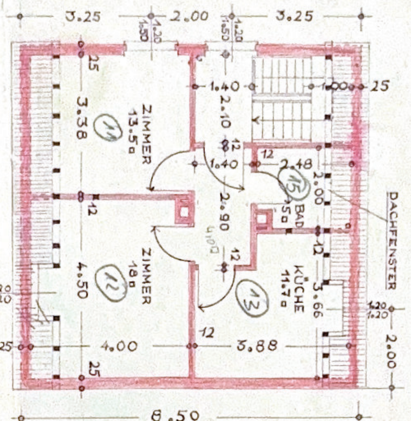
OBERGESCHOSS
