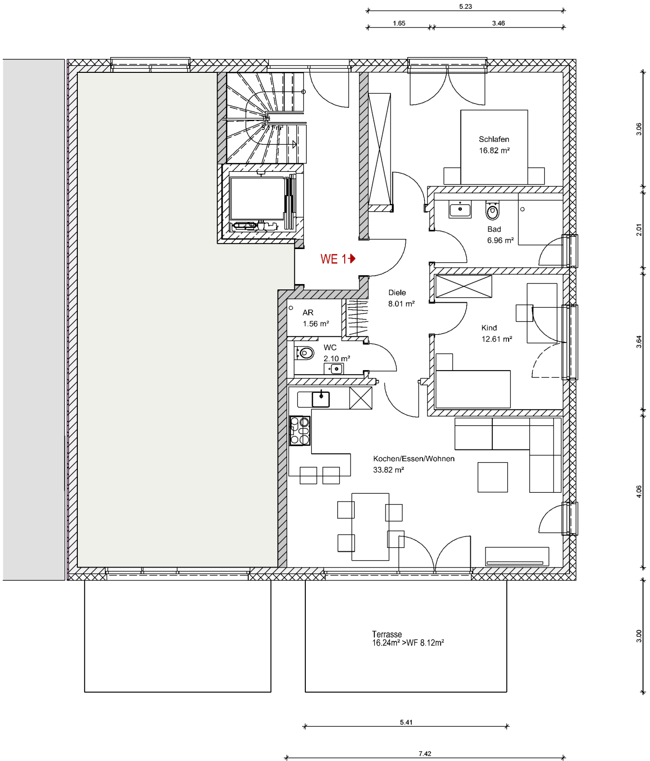
Wohnung WE 1_EG links
