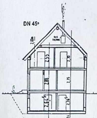
Schnitt
