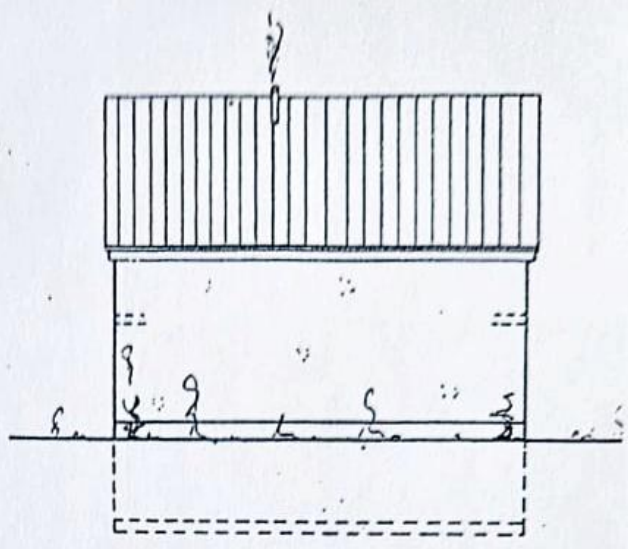
Ansicht – Nord-West
