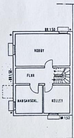
Kellergeschoss
