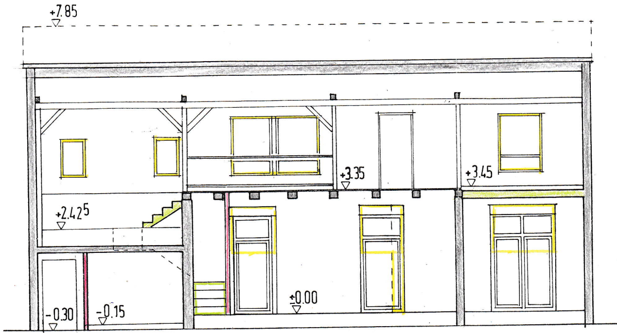
SCHNITT 1-1
