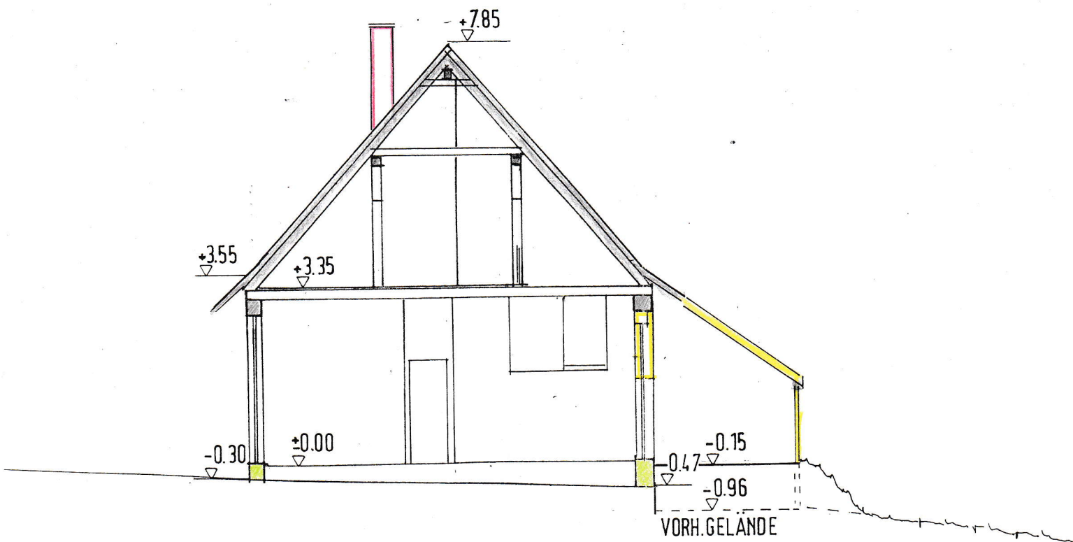
SCHNITT 1-1
