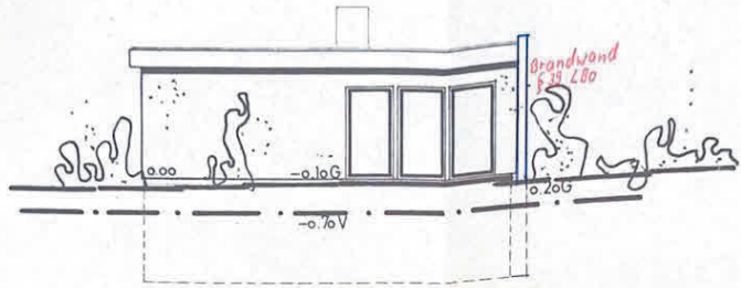
SEITENANSICHT RECHTS
