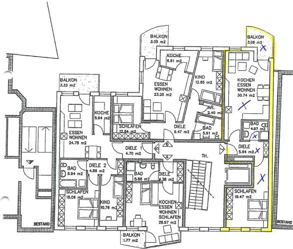
2. OBERGESCHOSS M 1/150
