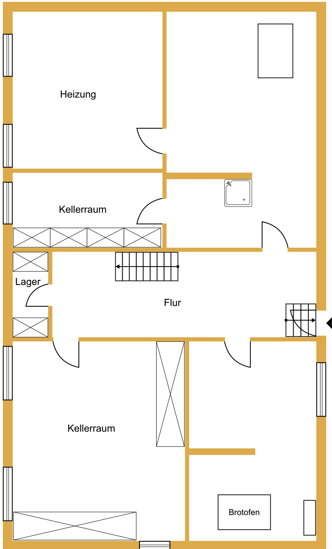
Kellergeschoss
