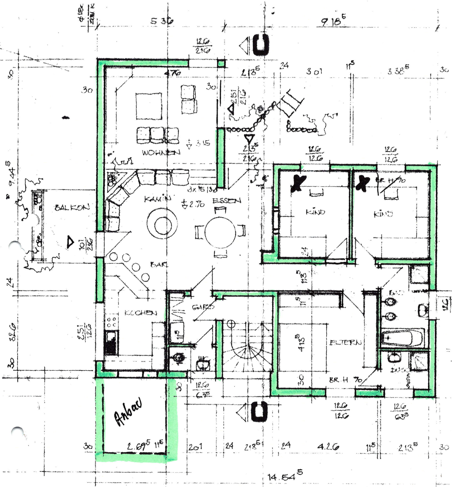
OBERGESCHOSS M 1:100
