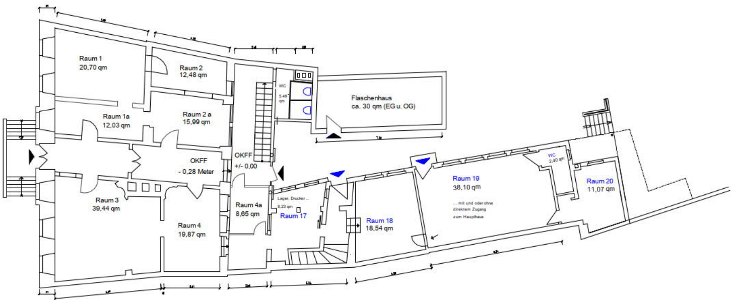
Erdgeschoss
