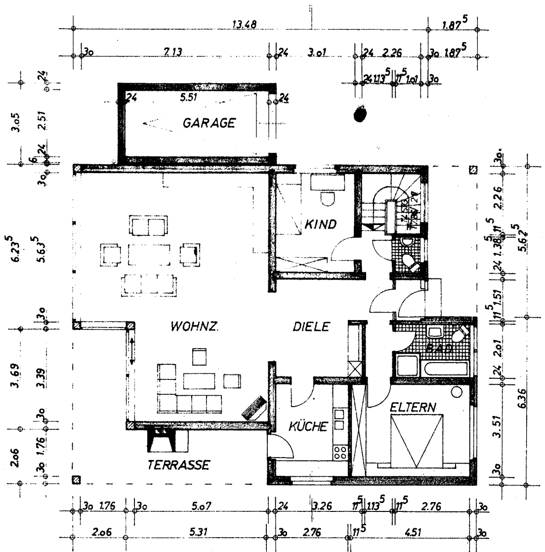
ERDGESCHOSS
