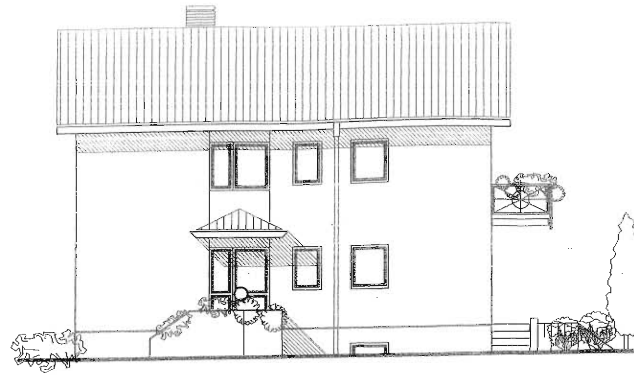
SÜDANSICHT
