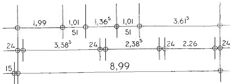
KELLERGESCHOSS M = 1 : 100
