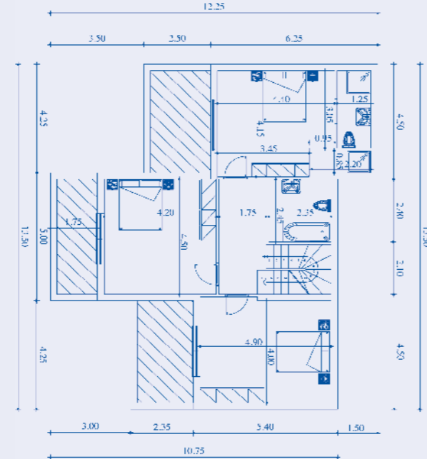
Grundriss: Obergeschoss
