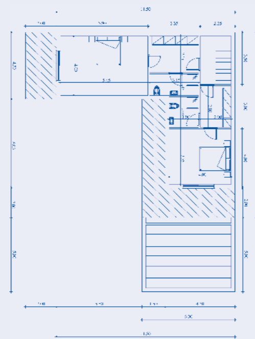
Grundriss: Obergeschoss
