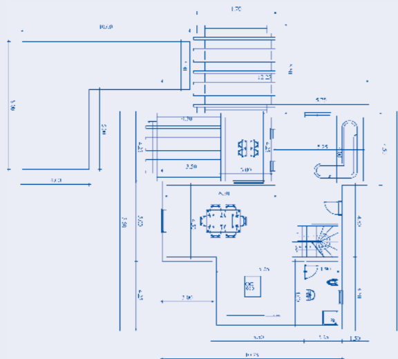
Grundriss: Erdgeschoss
